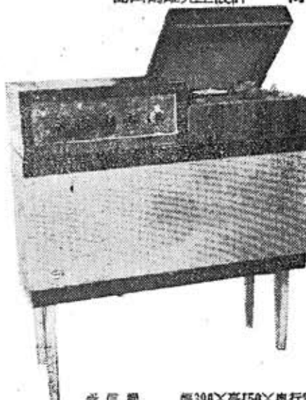
受信機 幅390×高150×奥行270mm プレーヤ 幅315×高150×奥行270mm SPボックス 幅705×高350×奥行270mm 脚高240mm
