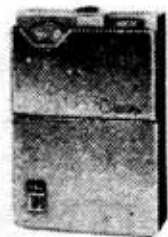
寸法 77×58×25mm
