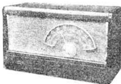
↓ハーモニー GS-52 型 寸法 476×275×215 mm RF なし 5〜6球 1B 用ダイヤル 6 \frac{1}{2} 〜7 \frac{1}{2} 用 ¥2,300.-
