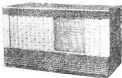
↑ニッカー NS-50 寸法 430×240×190 mm RF なし 5球スーパー用ナショナル型ダイヤル、オールネット 6 \frac{1}{2} 用 ¥1,250.-
