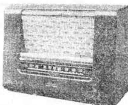
↑ハーモニー CD-2 型 寸法 450×330×220 mm RF なし 5球 1B 2B 用横行ダイヤルつき、適合スピーカー 6 \frac{1}{2} 〜7 \frac{1}{2} 用 ¥2,100.-
