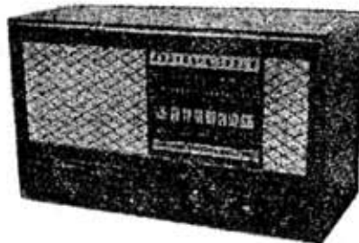
↑ クライスラー S 203 型 寸法 435×250×215 mm RF なし 5 球 1B 2B 用横行ダイ アルつき、適合スピーカー 6 \frac{1}{2} " 用 ¥1,480.-
