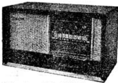
↑ トーヨー PR-1001 型 寸法 440×250×230 mm RF なし 1B 5 球スーパー用、 ブッシュボタンつき ¥3,050.-
