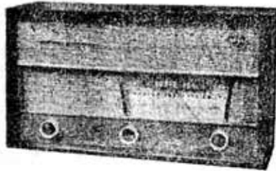
↑ クライスラー S 250 寸法 435×325×220 mm 5 球 1B 用横行ダイヤルつき、使用 スピーカー 6 \frac{1}{2} "~7" 用 マジック窓付 ¥1,750.-
