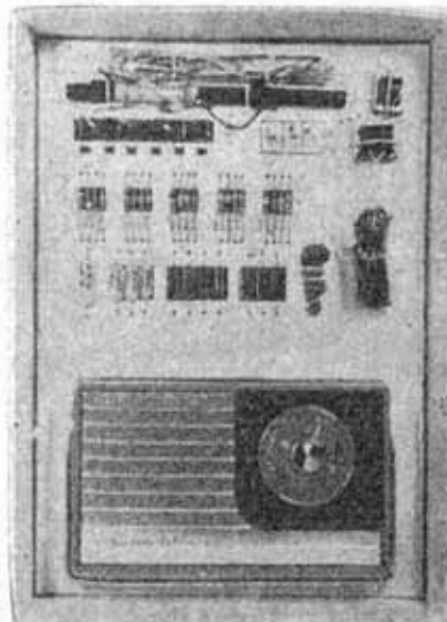
TRK-600 7,475円 6石トランジスタ・スーパーラジオ トランジスタ HJ-23, HJ-54×2 HJ-17, HJ-50×2 ダイオード SD-46
