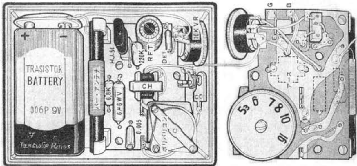
<上図はTRK-100の実体配線図です>
