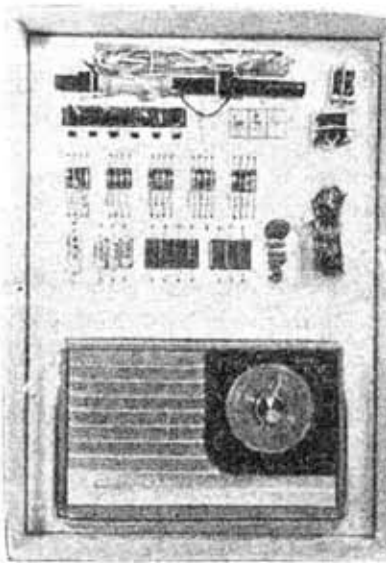
TRK-600 7,475円 6石トランジスタ・スーパーラジオ トランジスタ HJ-23, HJ-54×2 HJ-17, HJ-50×2 ダイオード SD-46
