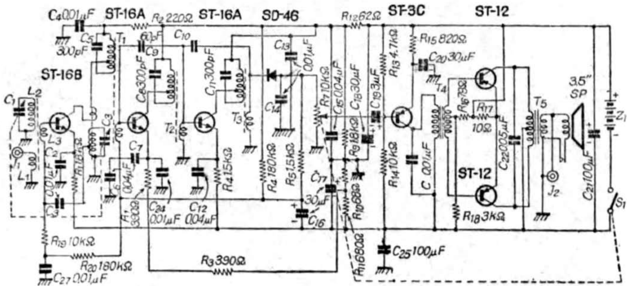
日本電気 NT6A の配線図
