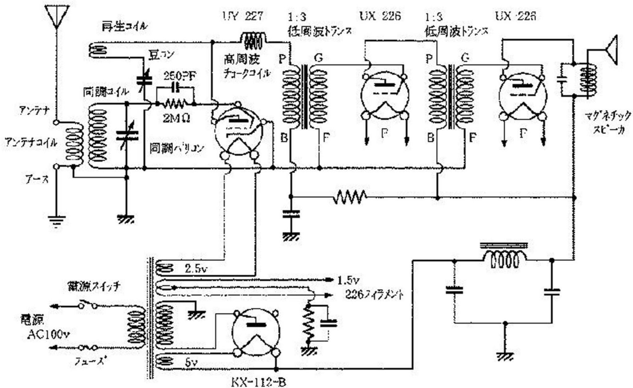
高島屋ダノン 再生式 4球エリミネータ受信機 回路図
