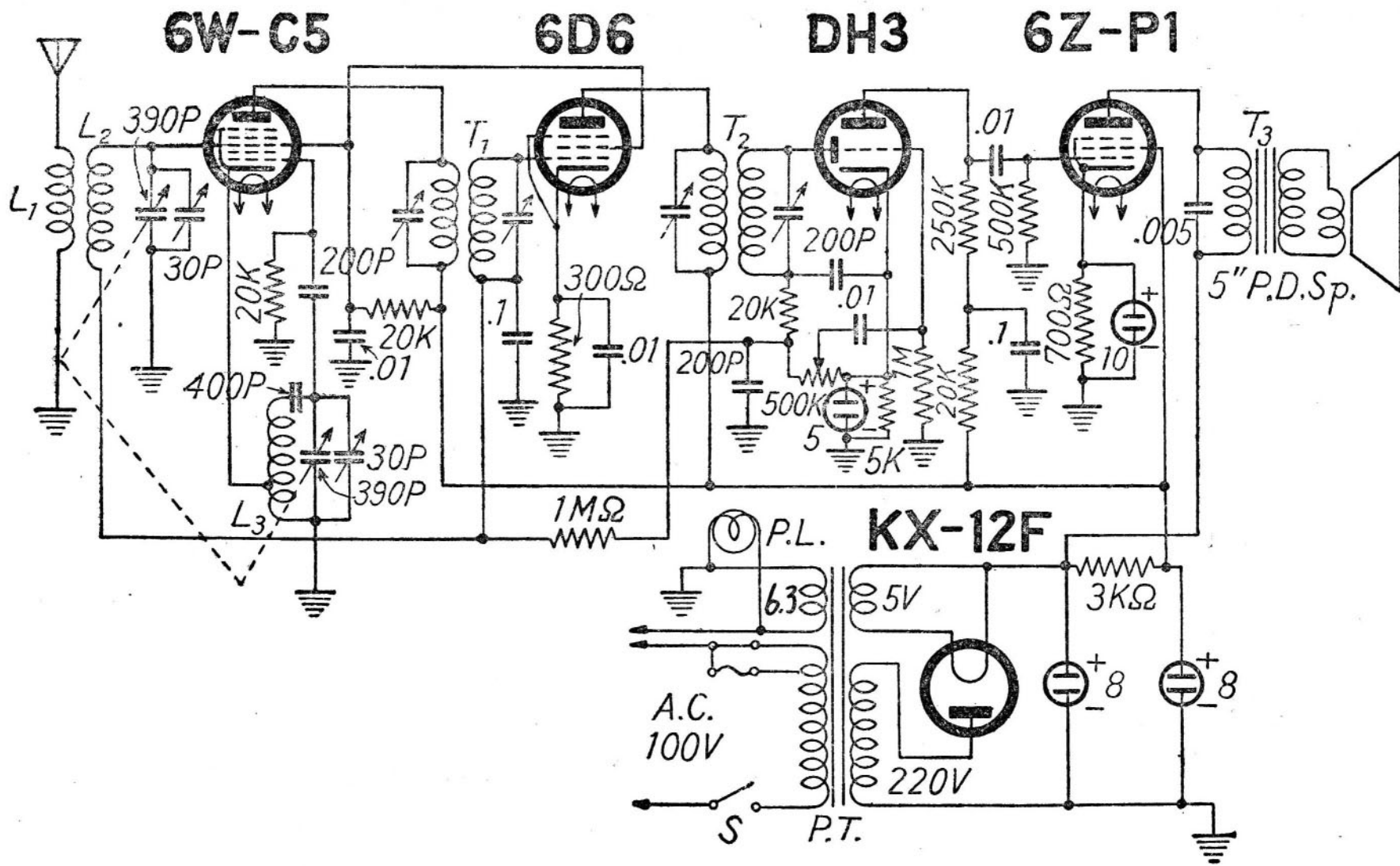
安立電機アルファA320型5球スーパー
