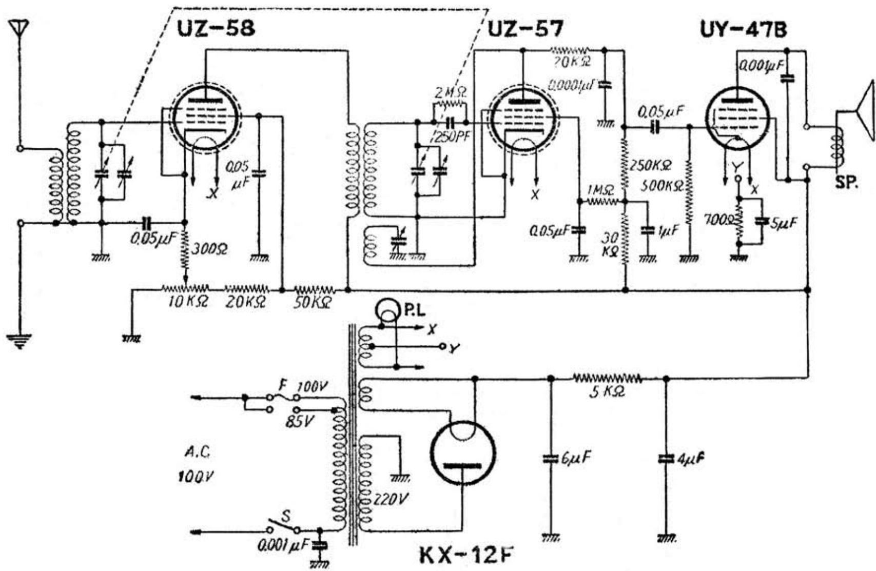
安立電機株式会社 (アルファ A-100 型) 国民 2 號型受信機
