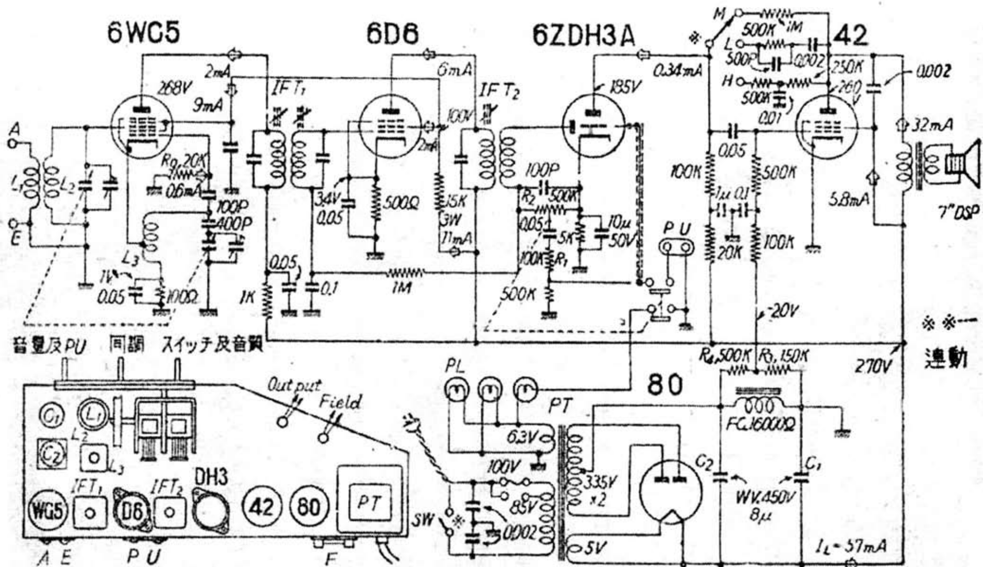
アリア DS-53B 型回路図
