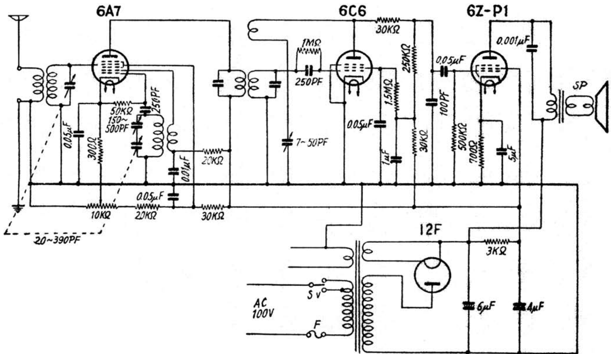
帝國電波〔クラリオン SD-4型〕
