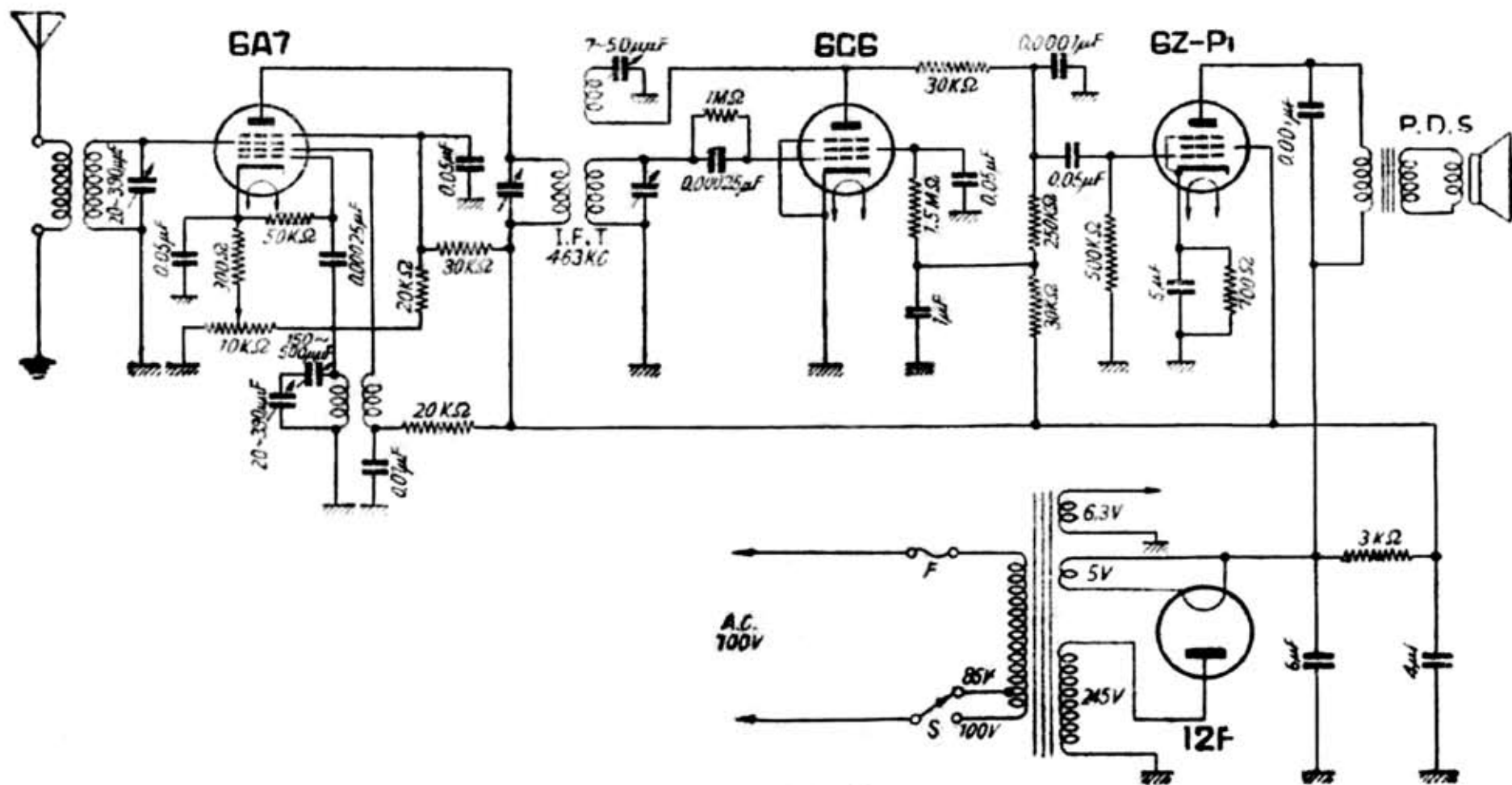
帝國電波型【クラリオンSD-4型】
