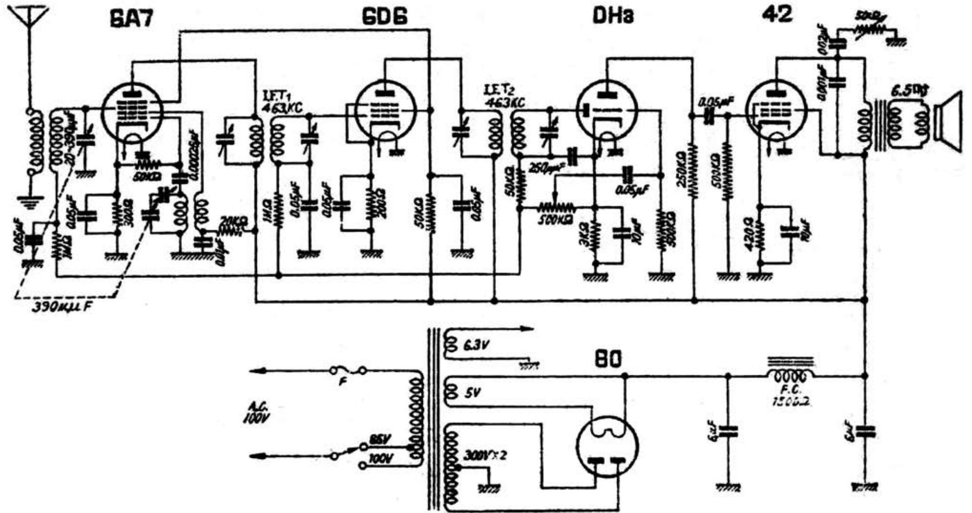
帝國電波製 クラリオンSD—5型] 5球スーパーヘテロダイン受信機
