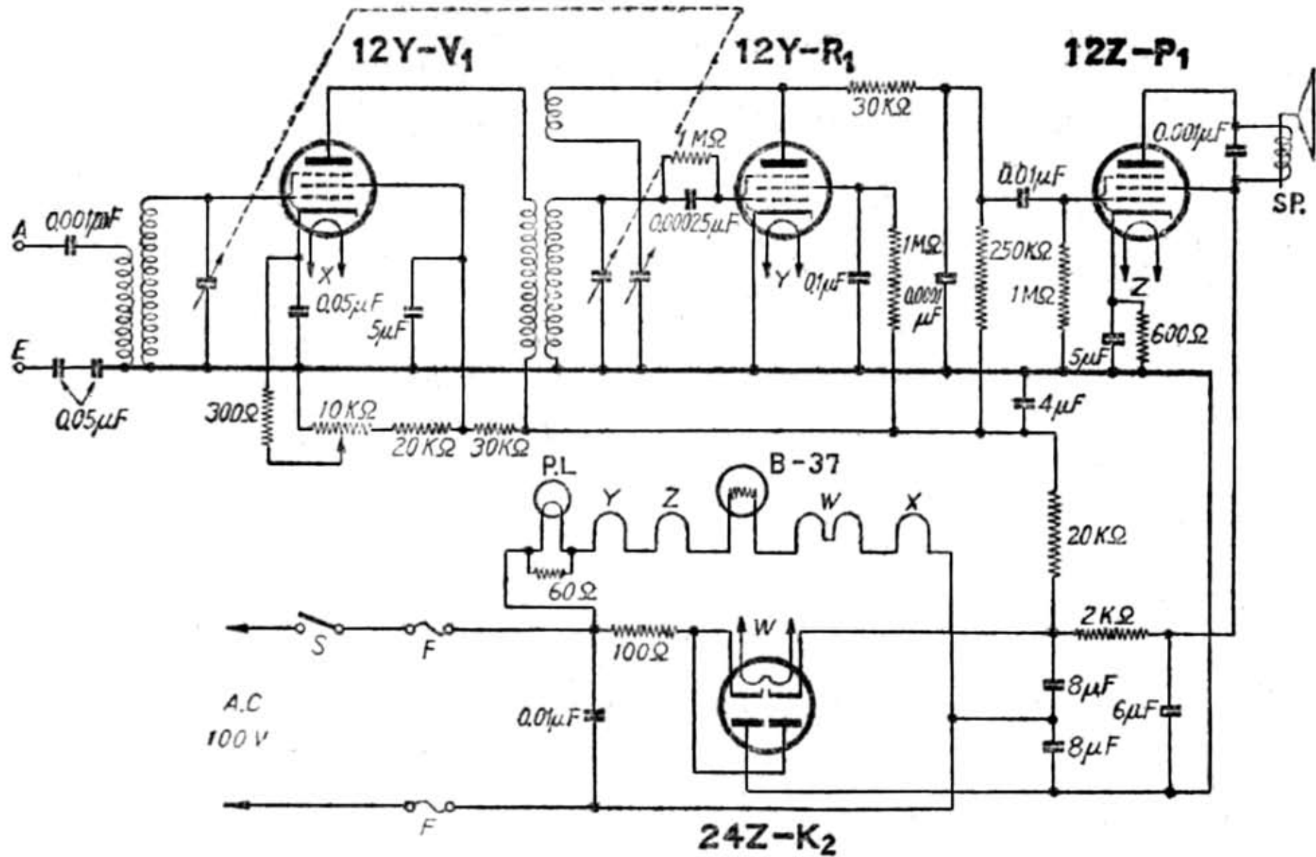
帝國電波株式會社 (クラリオン) 國民1號型受信機
