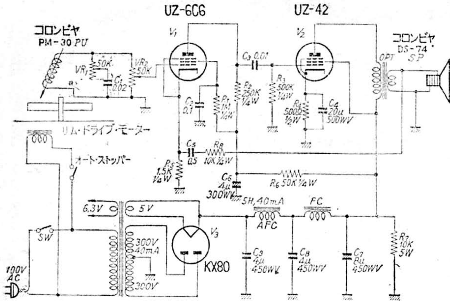
コロンビア EG-38 型の回路
