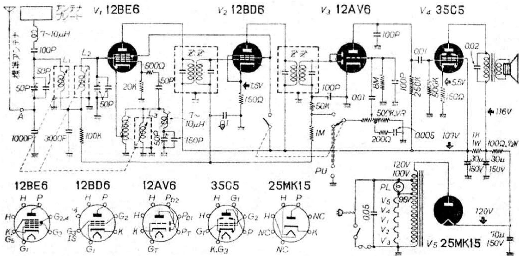
コロムビア R-541 回路図
