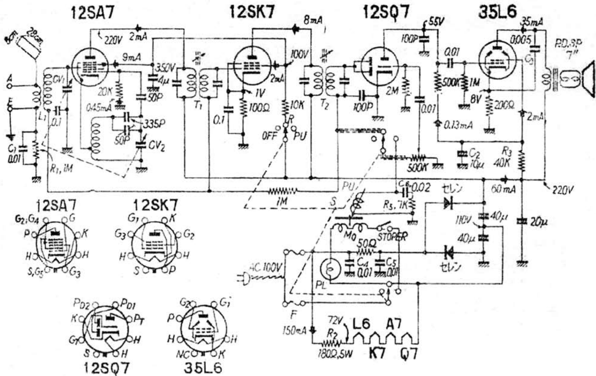
コロムビア RG-510 型電蓄回路図
