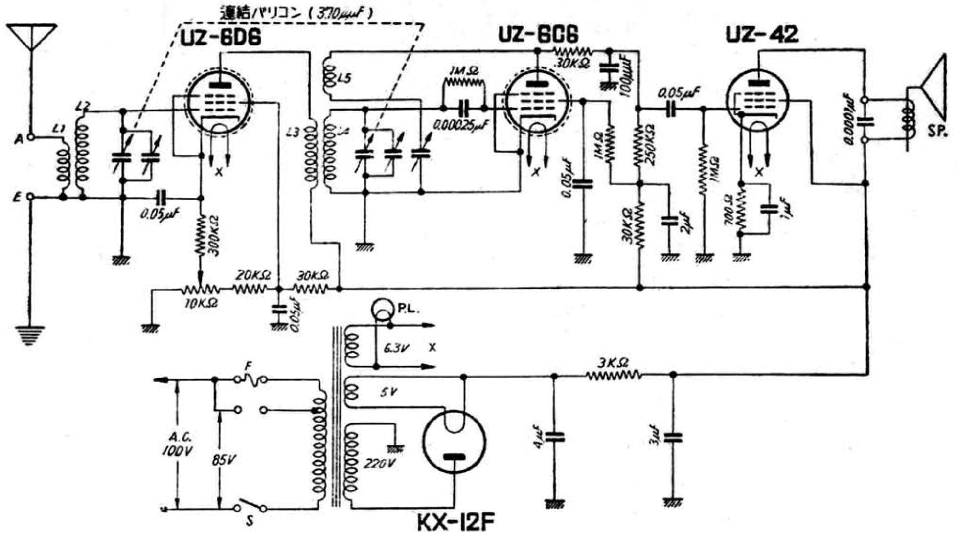
戸根無線製 [コンサートン] 國民2號 C型受信機
