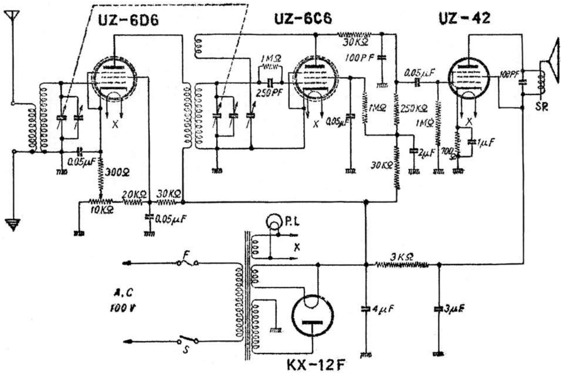
戸根無線株式会社 (コンサートン) 國民 2 號型受信機
