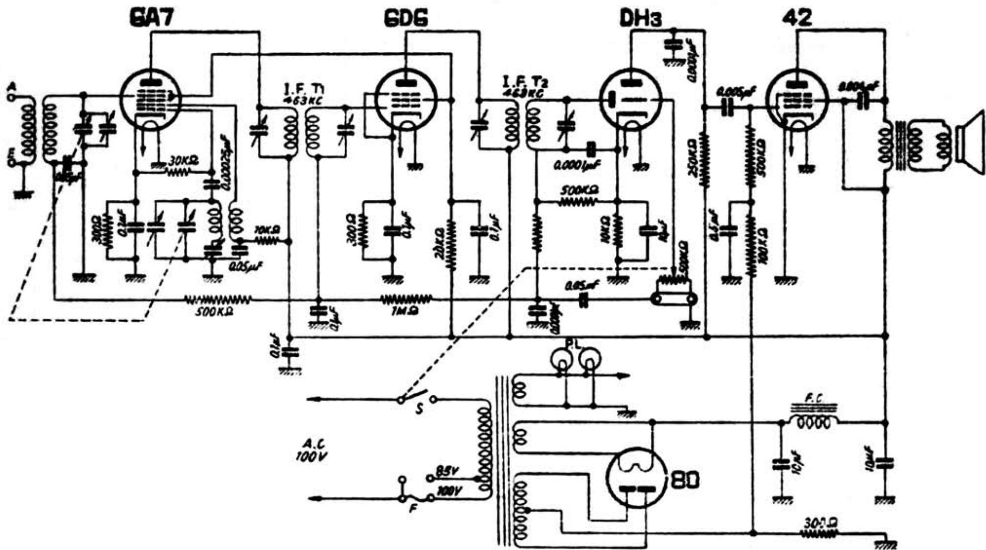
日本精器製〔クラウン CR-5S1型〕5球スーパーヘテロダイン受信機
