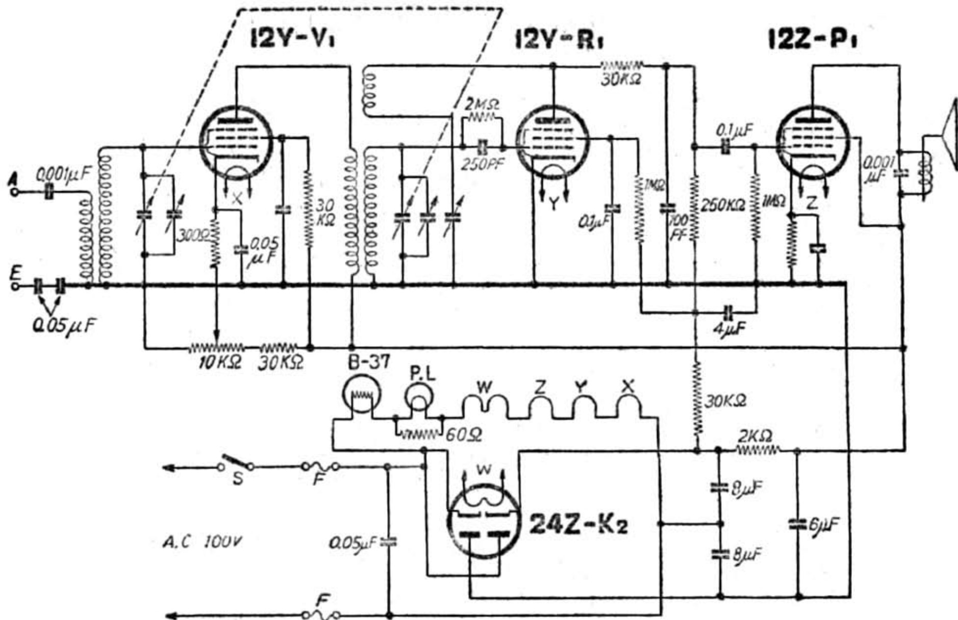
日本精器株式会社 (クラウン) 国民 1 号型受信機
