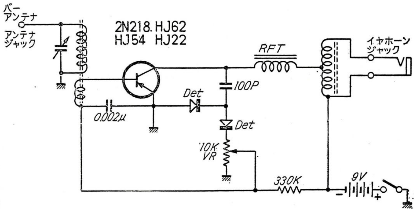
クラウン TR-11A 型
