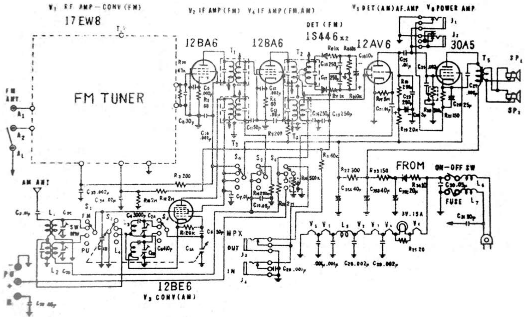
FM / AM RADIO TRV.- 352
