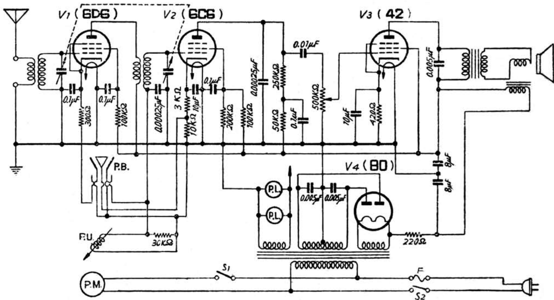
不二家フォン [PRT-101型] 卓上型ラジオ電気蓄音機
