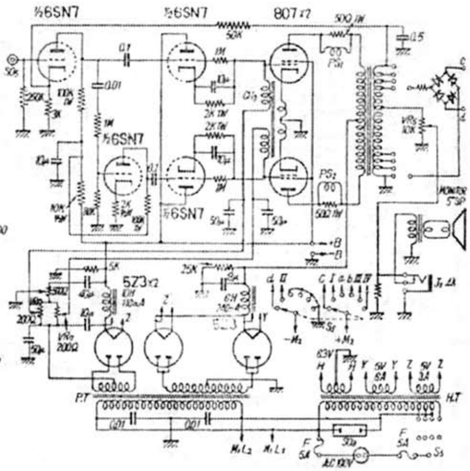
アンプ部
