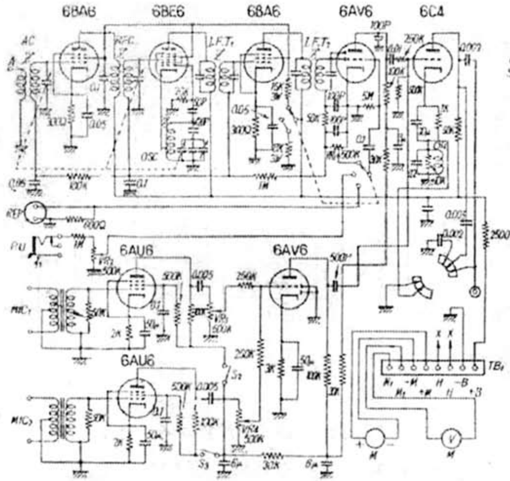
ラジオ部
