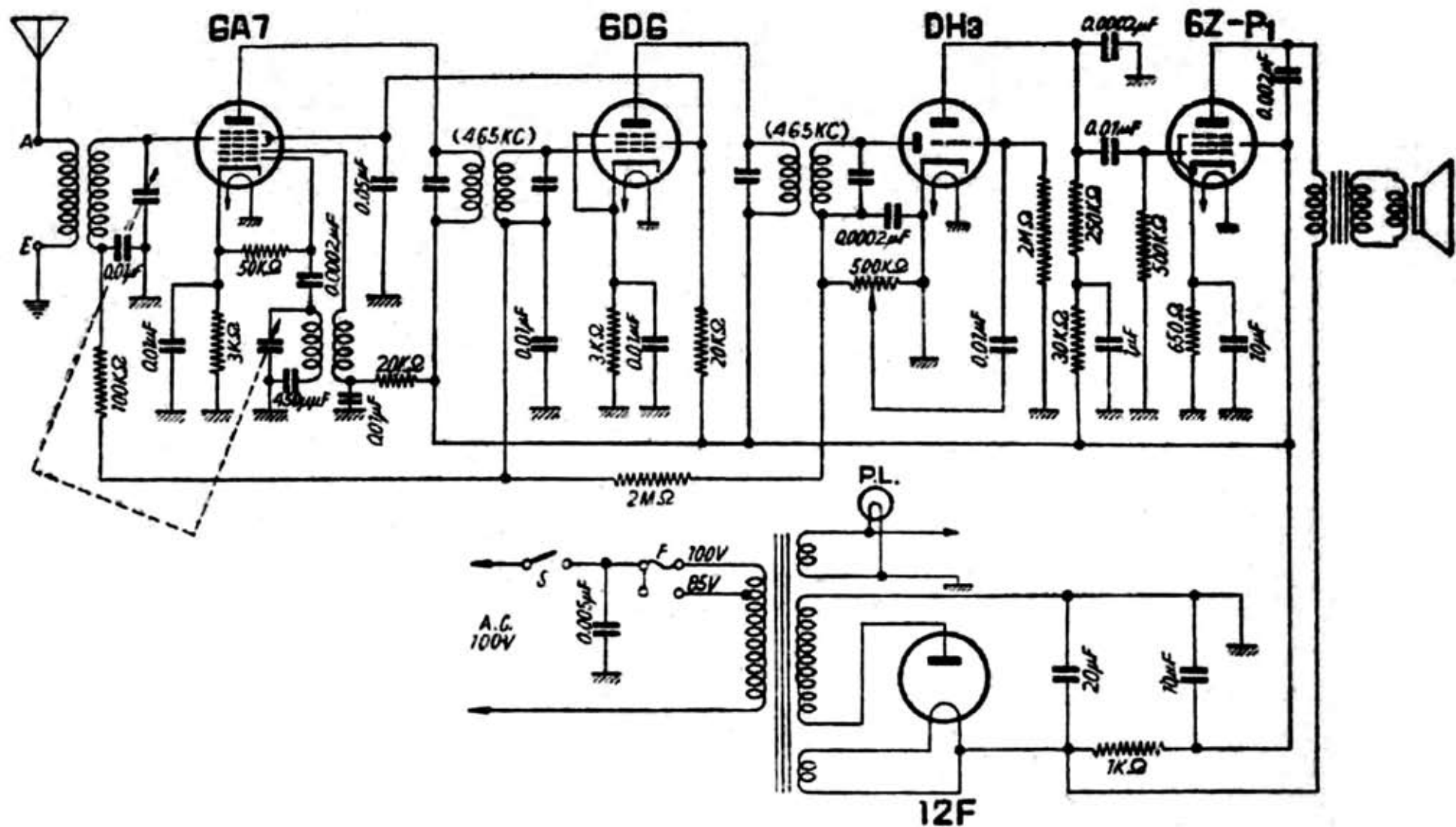
八歐無線電機 [ゼネラル 5NS-1型] 5球スーパーヘテロダイン受信機
