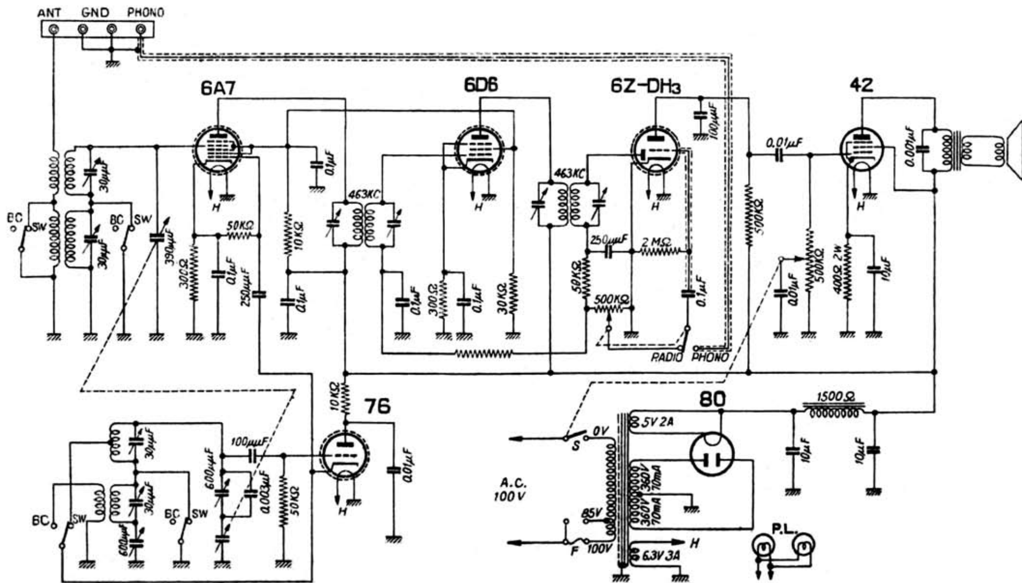
原口無線電機 [キャラバン D-660型] 6球2バンドスーパーヘテロダイン受信機
