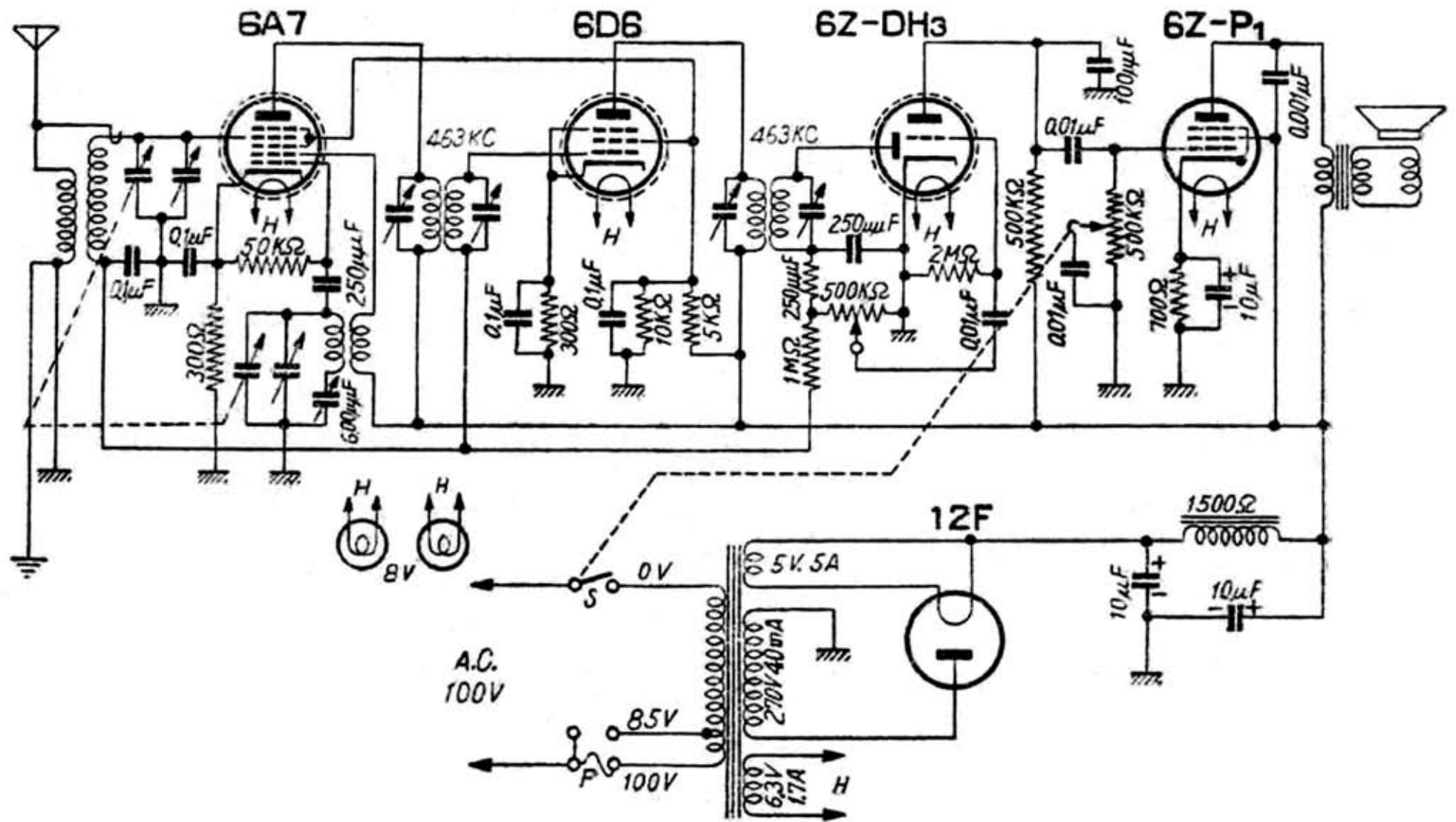
原口無線電機〔キャラバンド—95型〕5球スーパーヘテロダイン受信機
