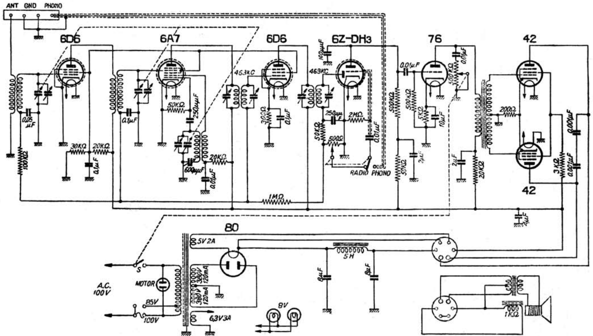
原口無線電機製 [キャラバン T-80型] 8球スーパー兼電気蓄音機
