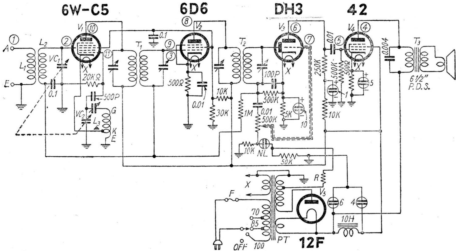
大阪ヘルメスS-52S型 5球スーパー
