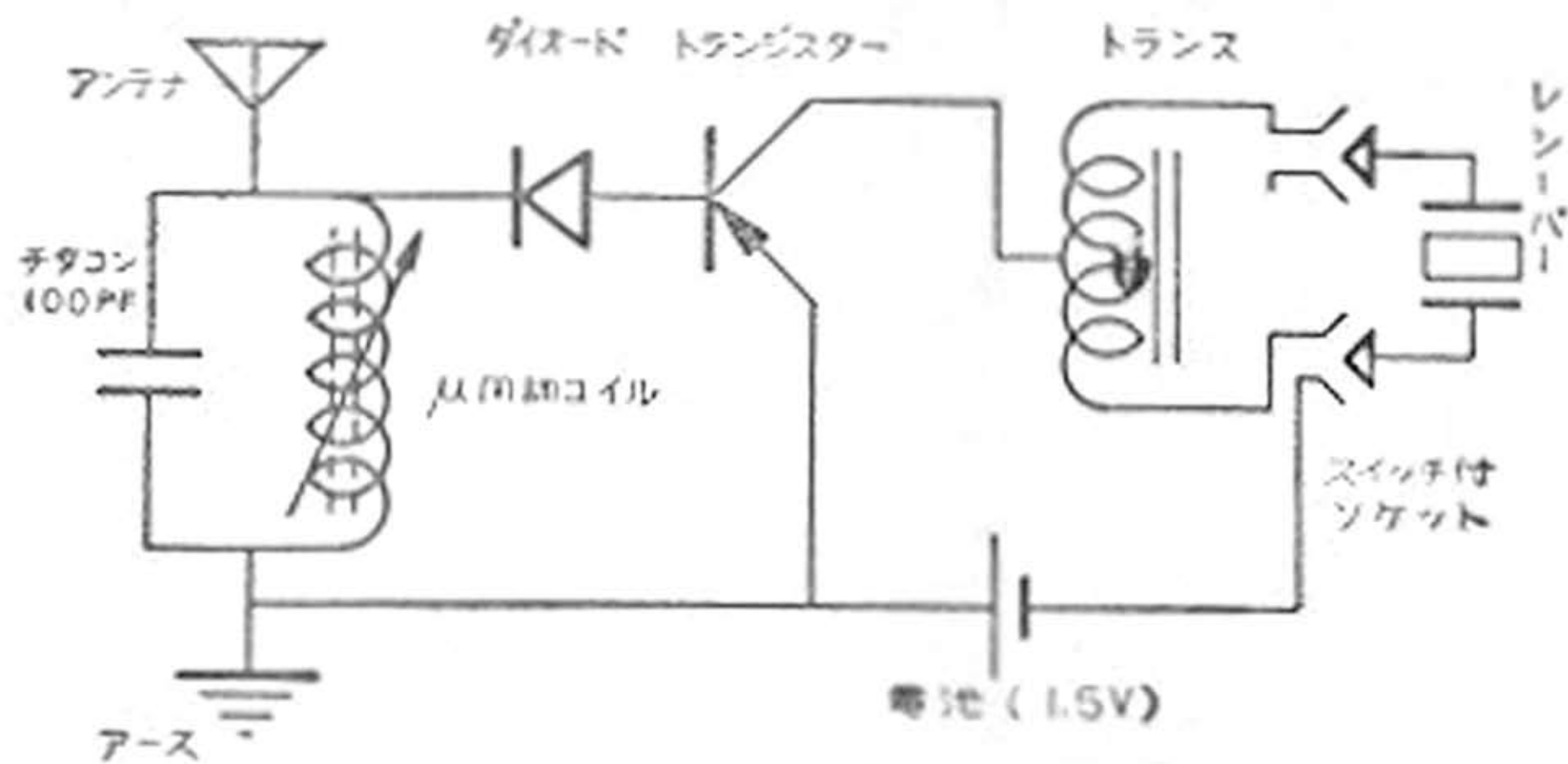
ヒノテ T-6 回路図
