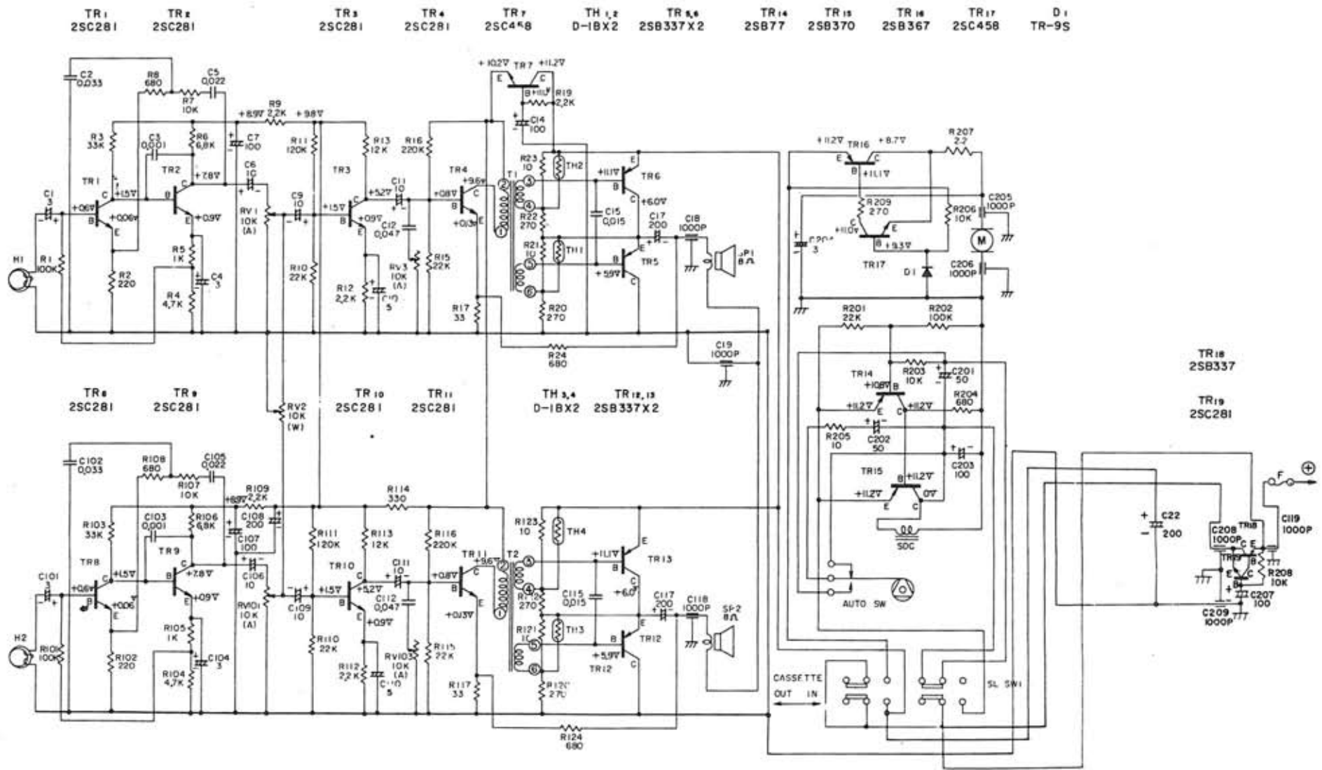
「日立」CS-203 回路図
