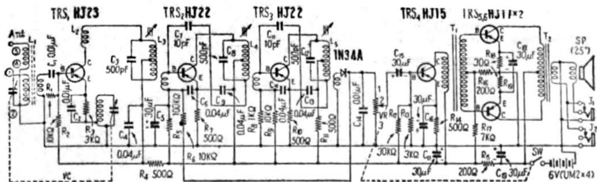
日立 TP690 の配線図
