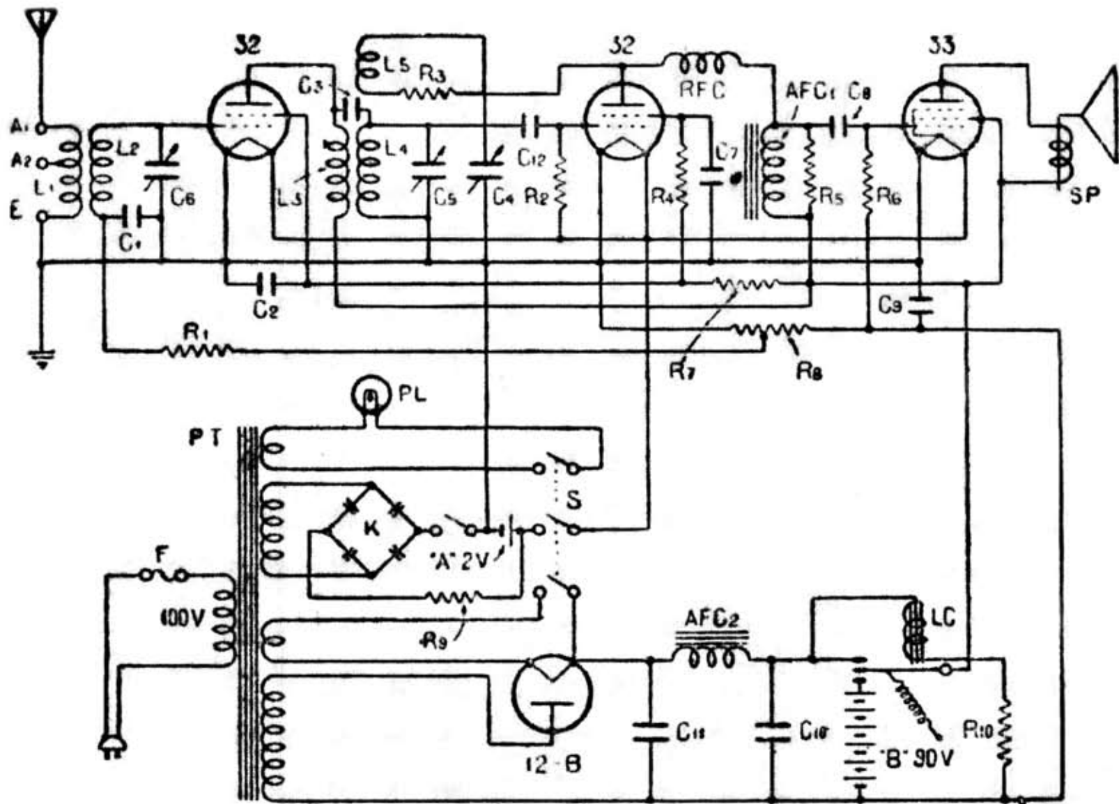
F-400型国防受信機の配線圖
