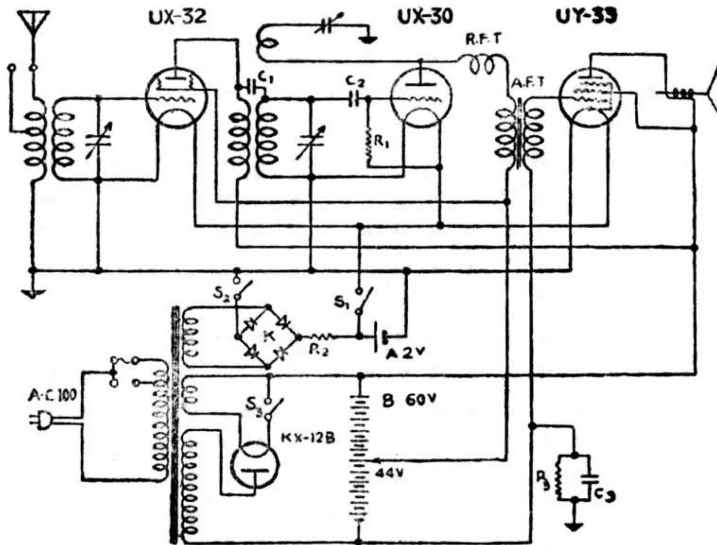
国防受信機 FB-4型国防受信機の配線圖
