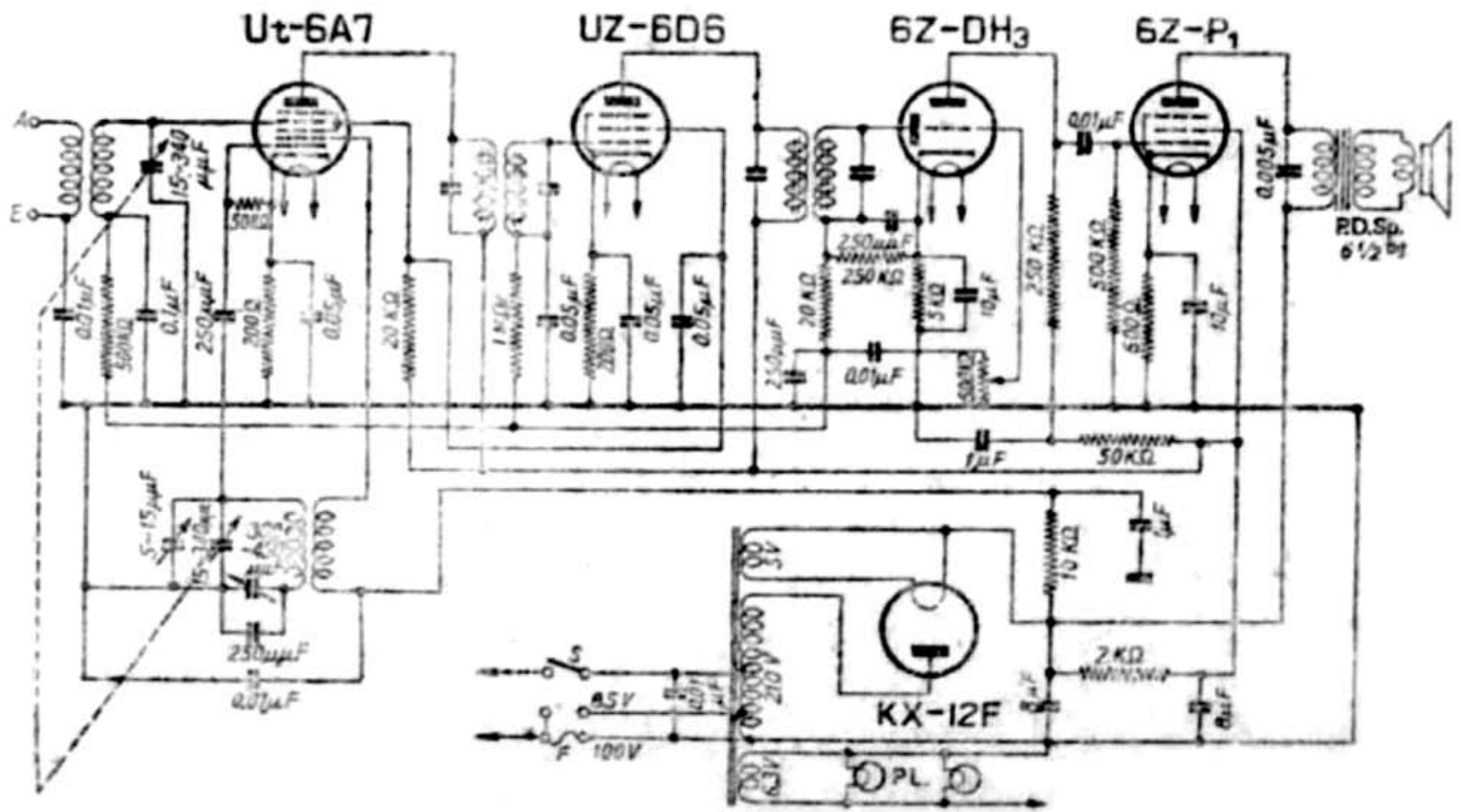
双葉電機製 國民型5球式スーパーヘテロダイン受信機
