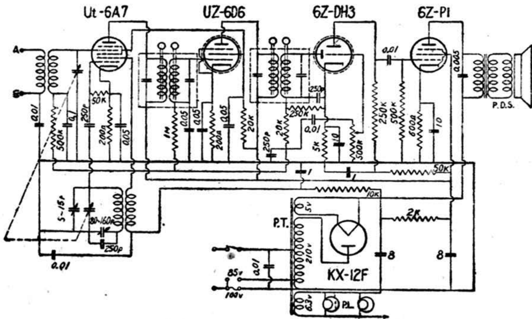
「双葉」普及型スーパー受信機 FKS 型
