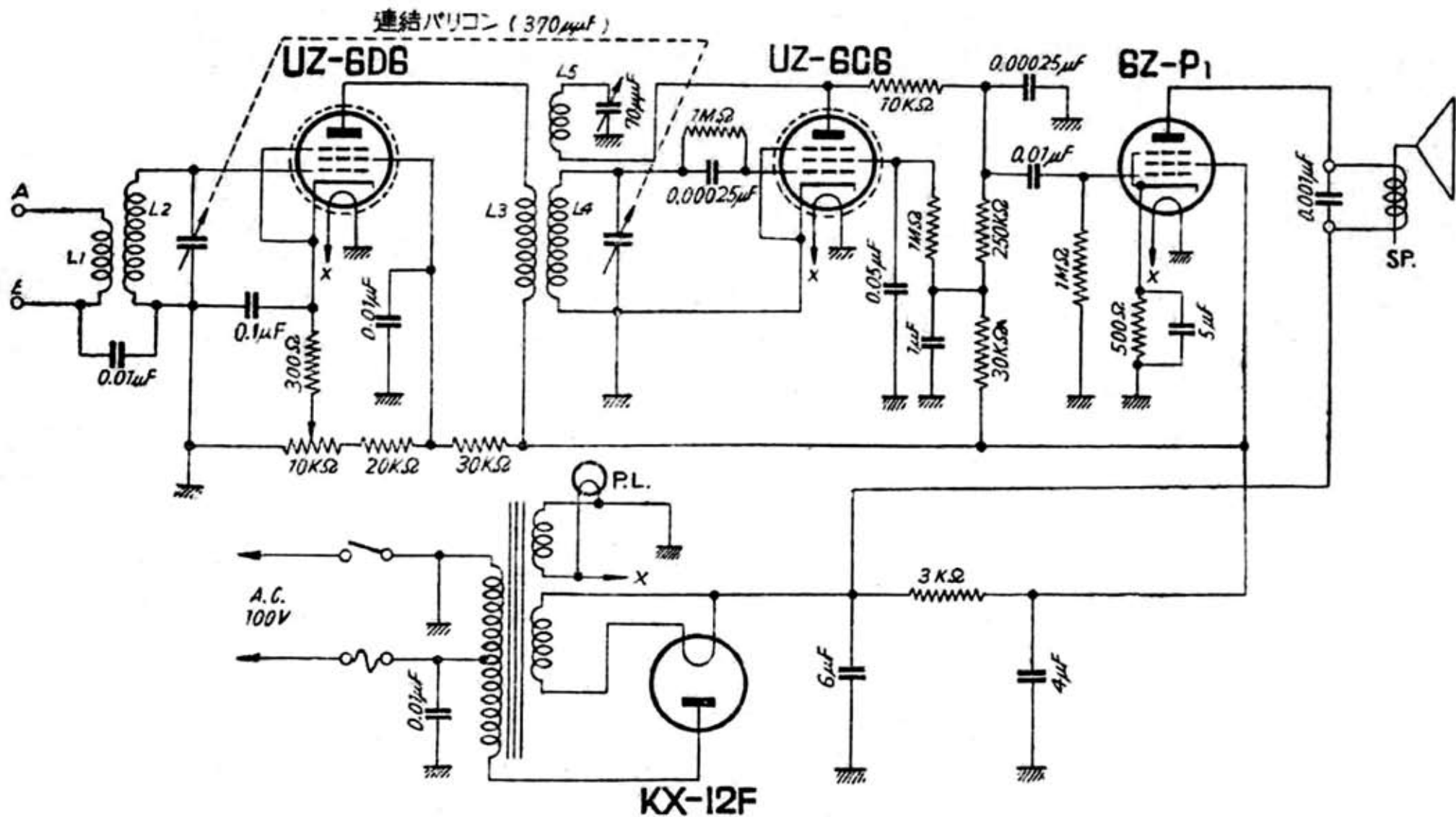
双葉電機製 [双葉] 國民2號A型受信機
