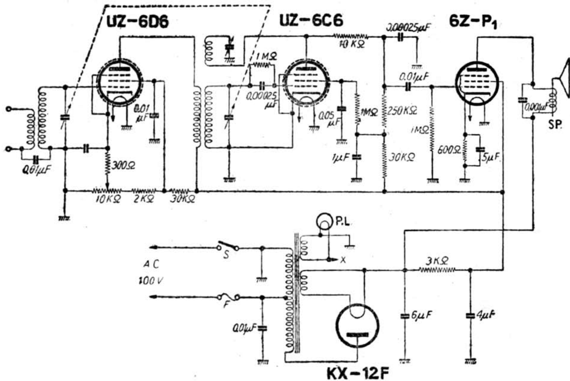
双葉電機株式会社（双葉）國民2號型受信機
