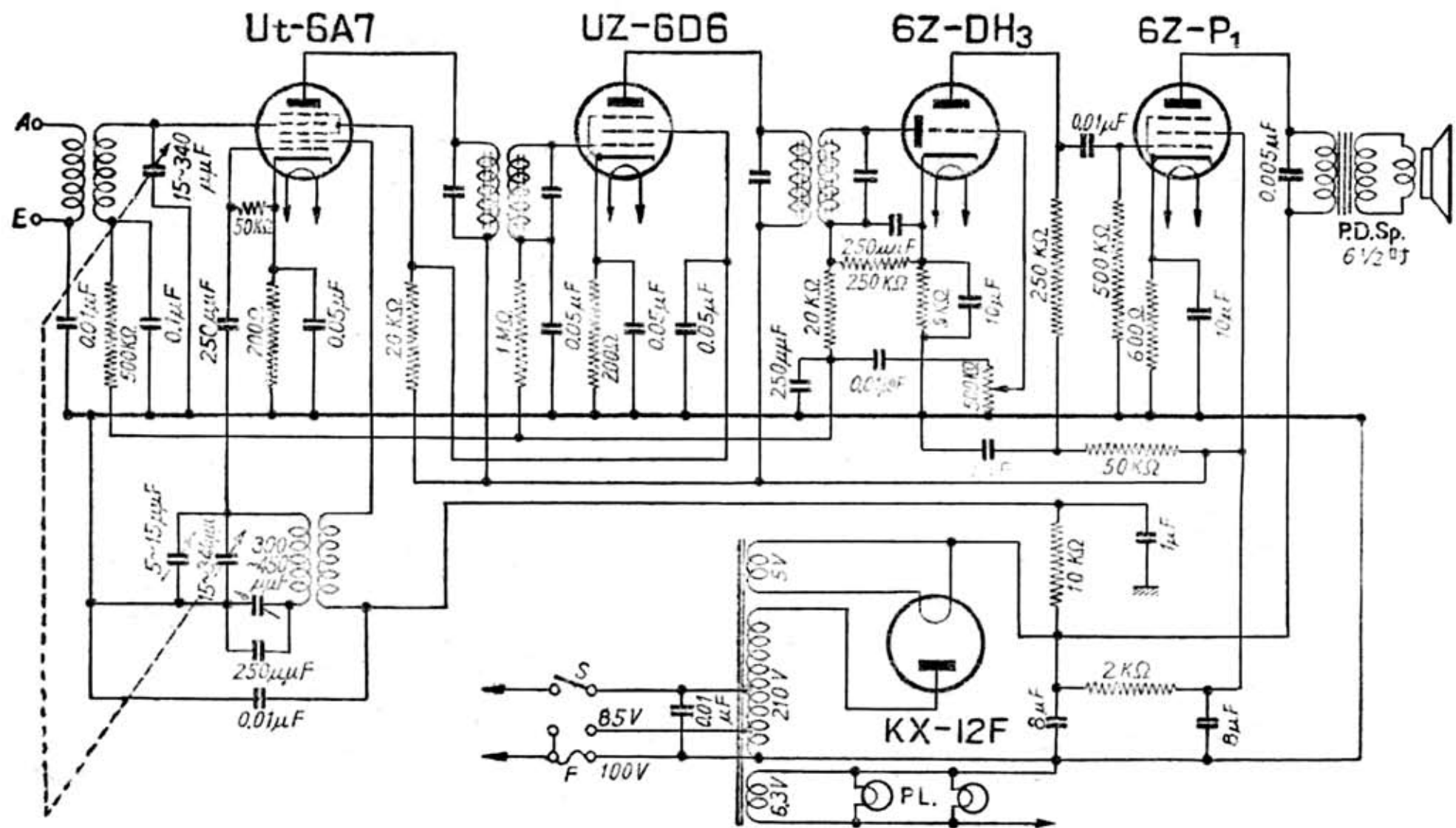
双葉電機製〔双葉〕スーパー100型国民型受信機
