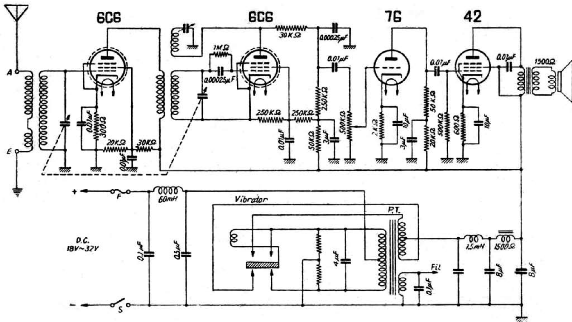
日本電子工業製 [ゼニック FV-1 型 漁船用直流受信機]
