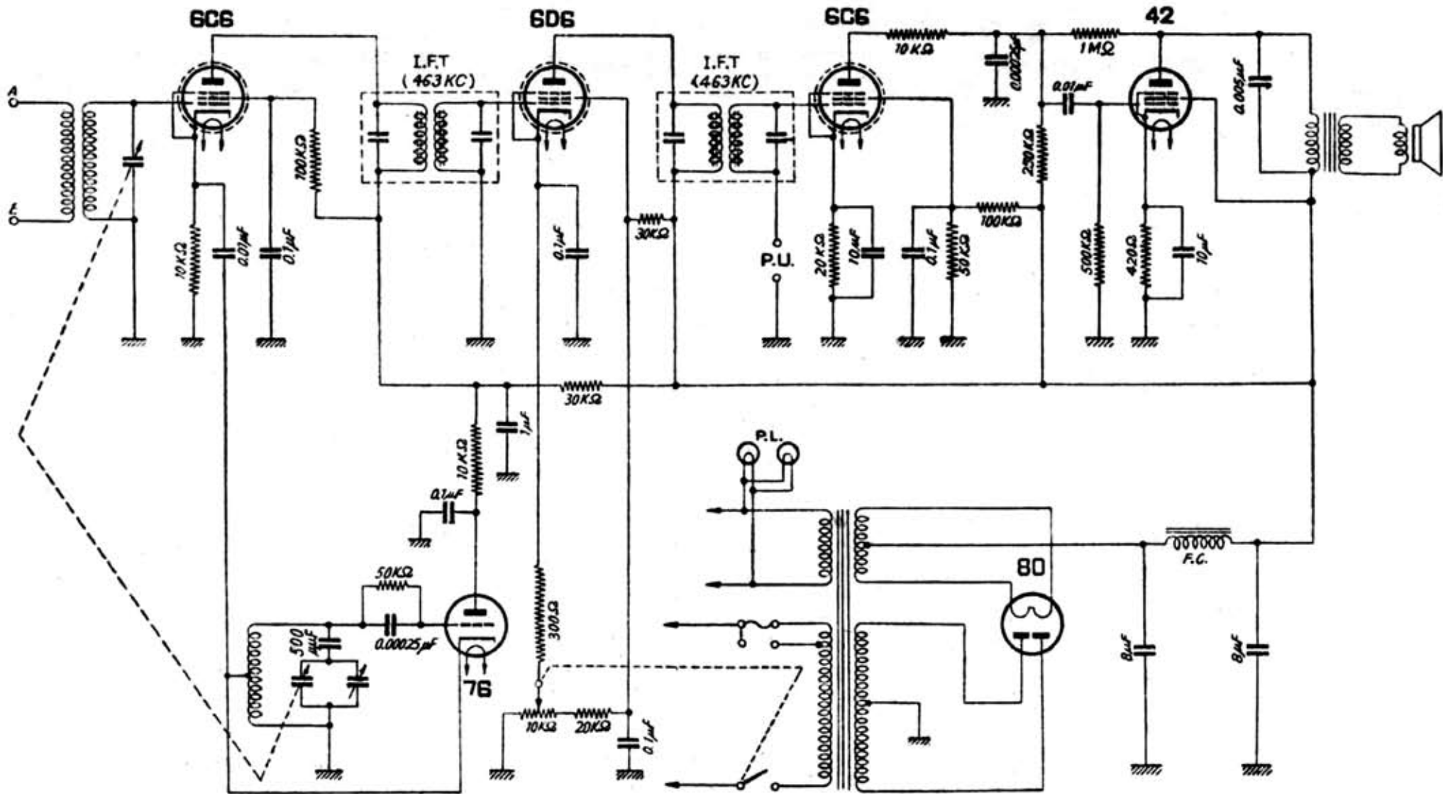
日本電子工業製 [ゼニック SB-500型] 6球スーパー受信機
