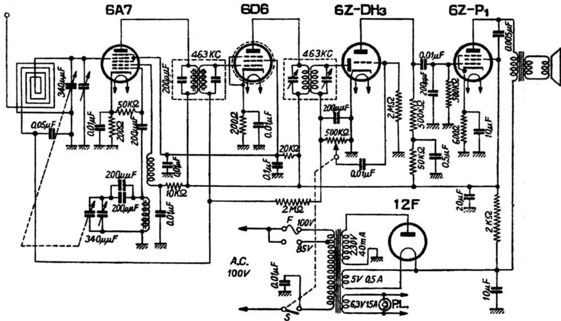
日本無線製「JRC NR-5A型」5球スーパーヘテロダイン受信機
