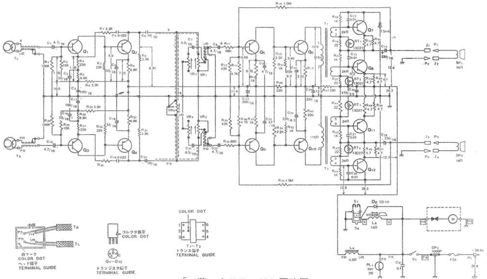
「三菱」ATP-424 回路図
