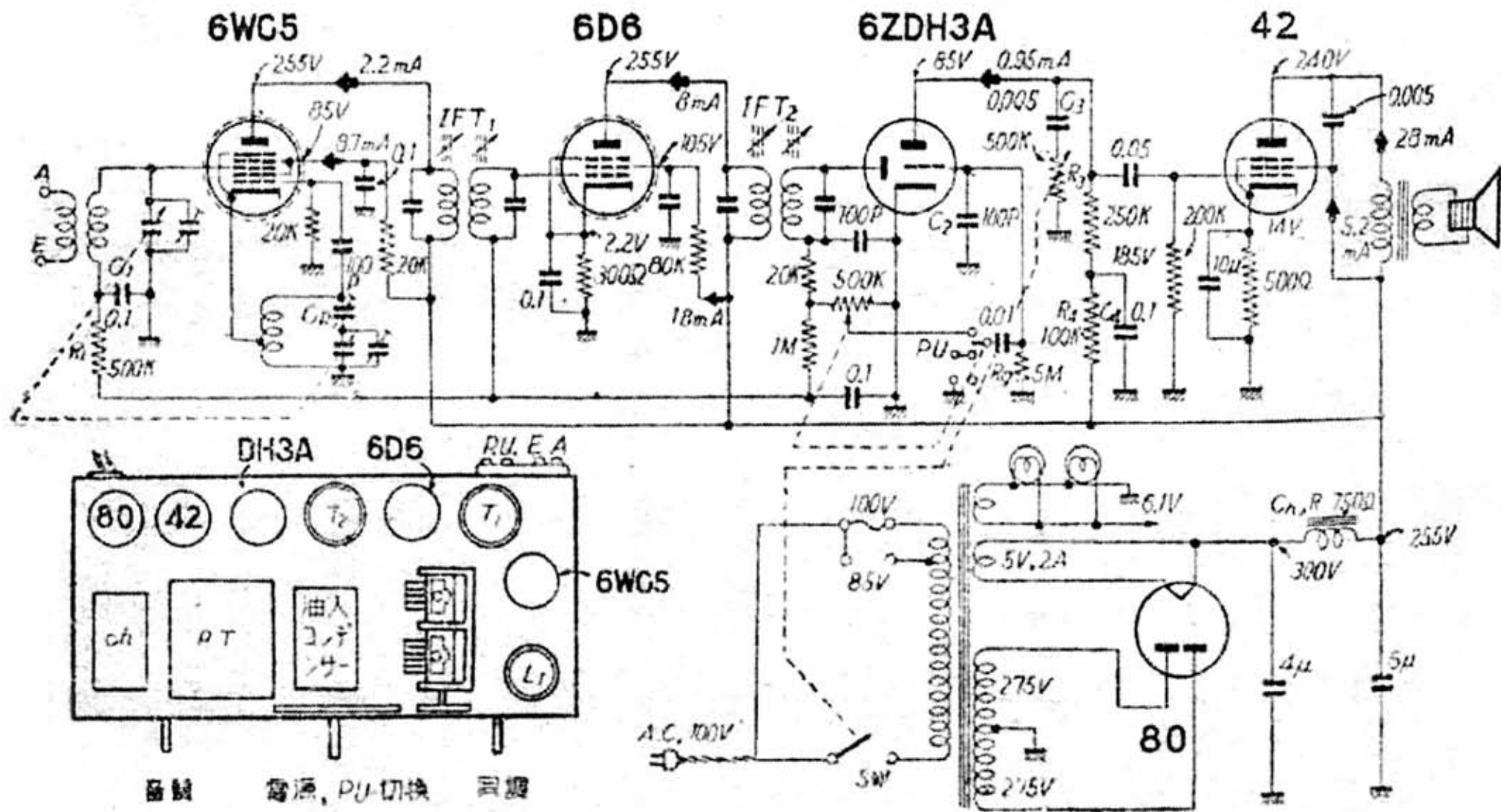
ダイヤトーン(三菱)M型5球スーパー
