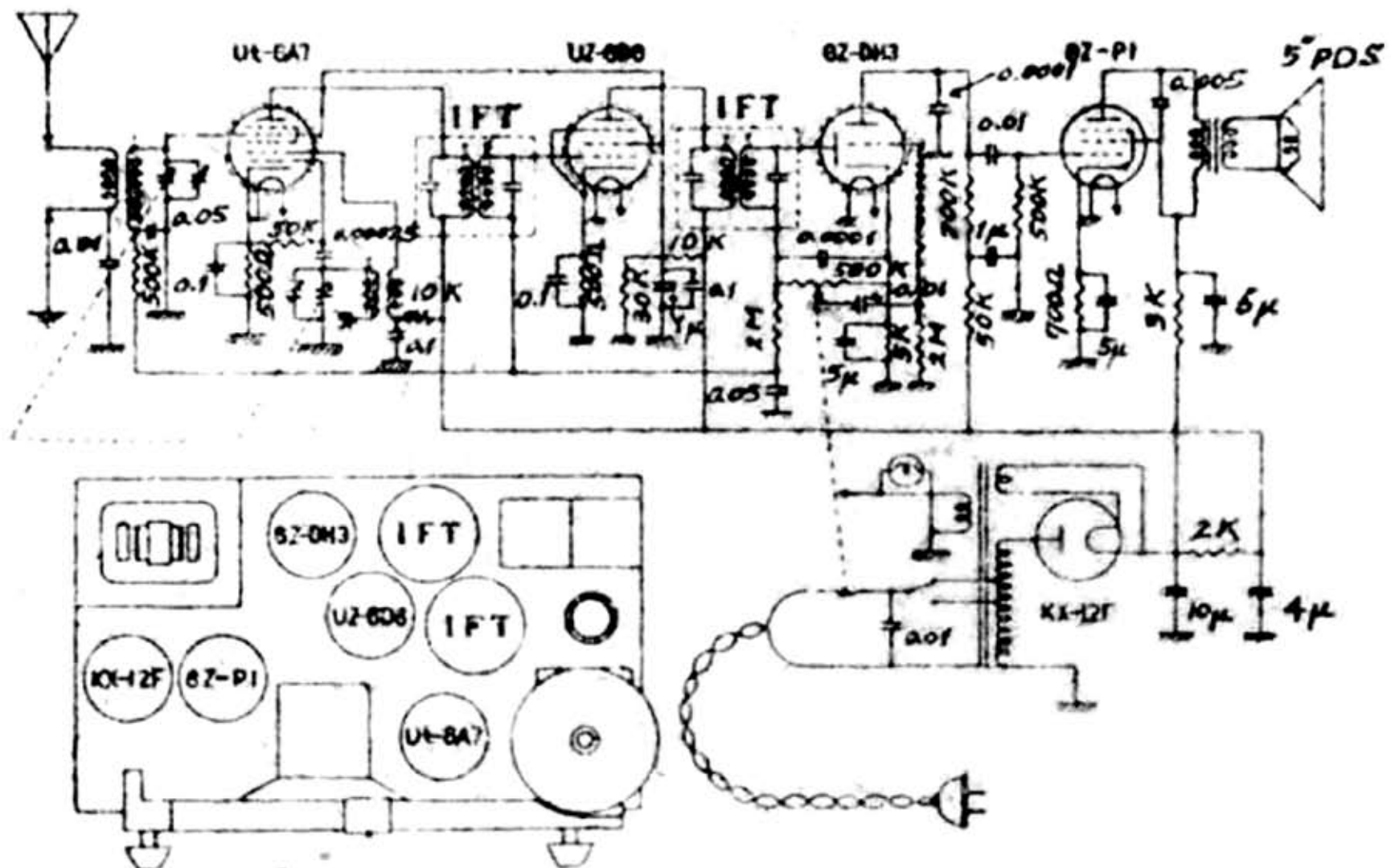
48-G 型ラジオ配線図並に配置図
