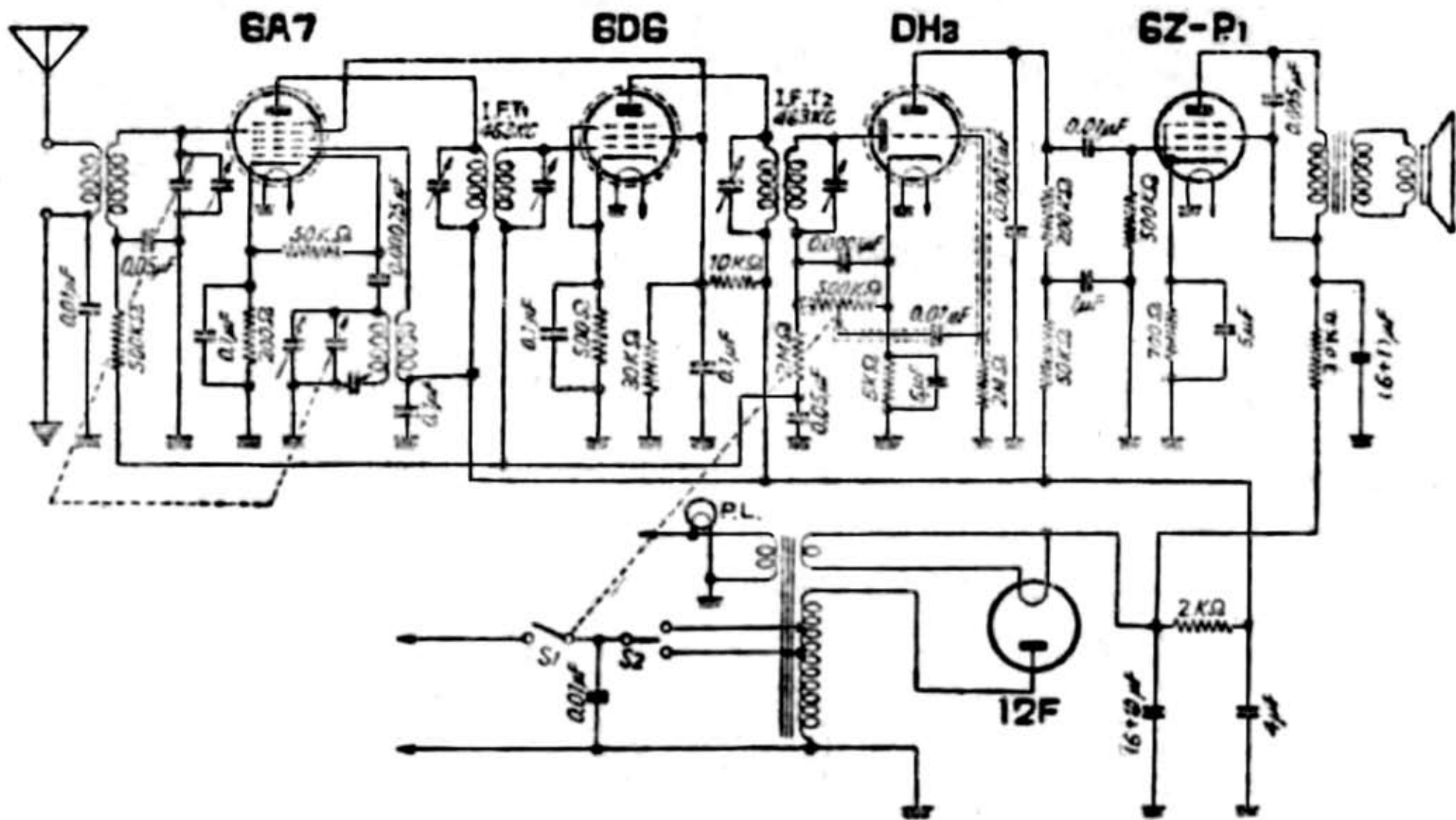
三菱電機製 ダイヤトーン 48-G 型 5 球式スーパーヘテロダイン受信機
