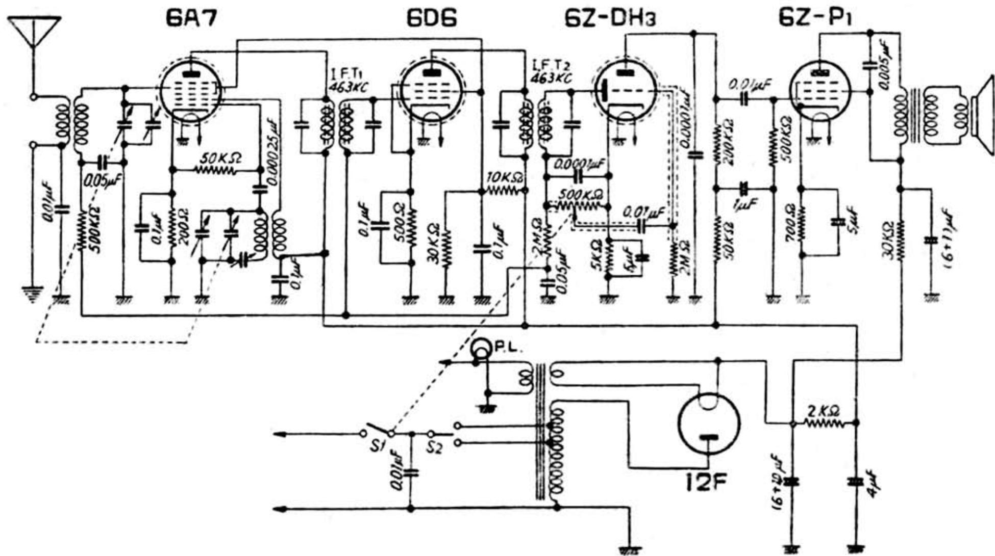
三菱電機製 [ダイヤトーン 48—G 型] 5 球スーパーヘテロダイン受信機
