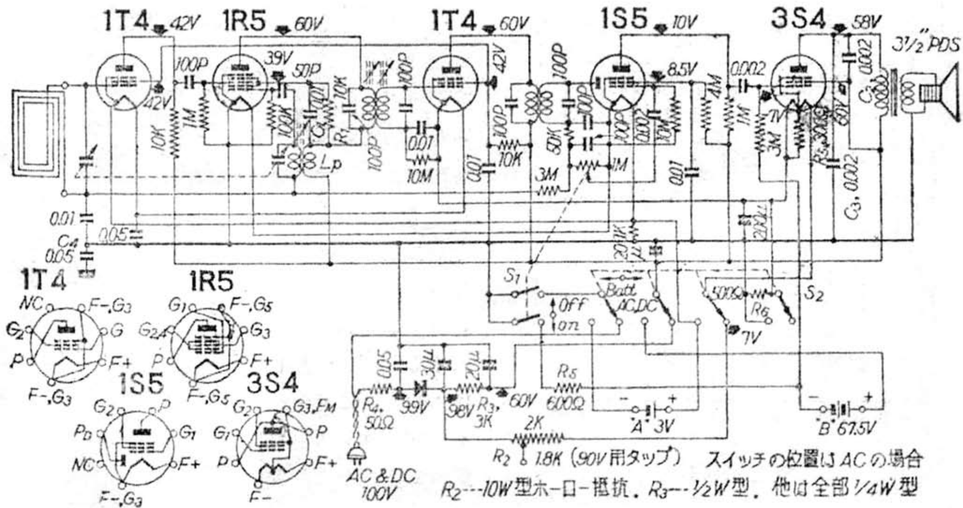
中島無線 F-125型 3 ウエイ・ポータブル受信機回路図
