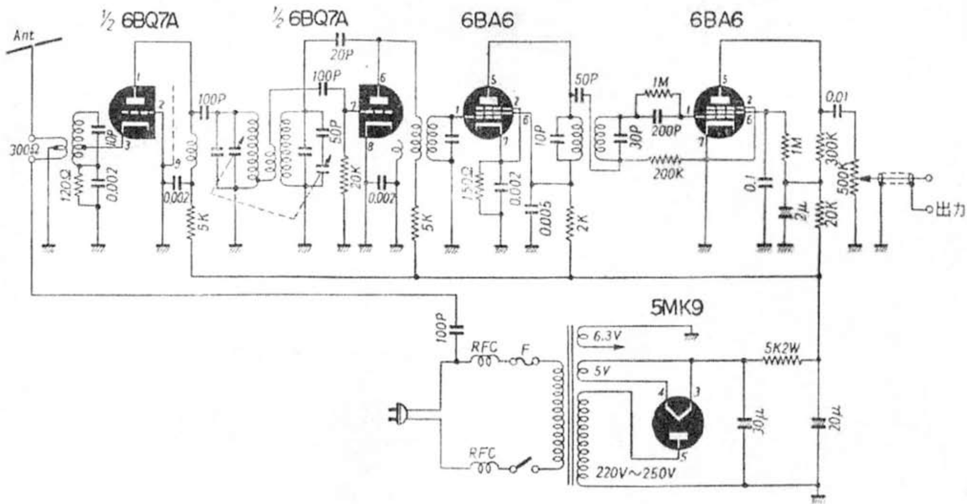
ナナオラ 簡易形FMチューナ
