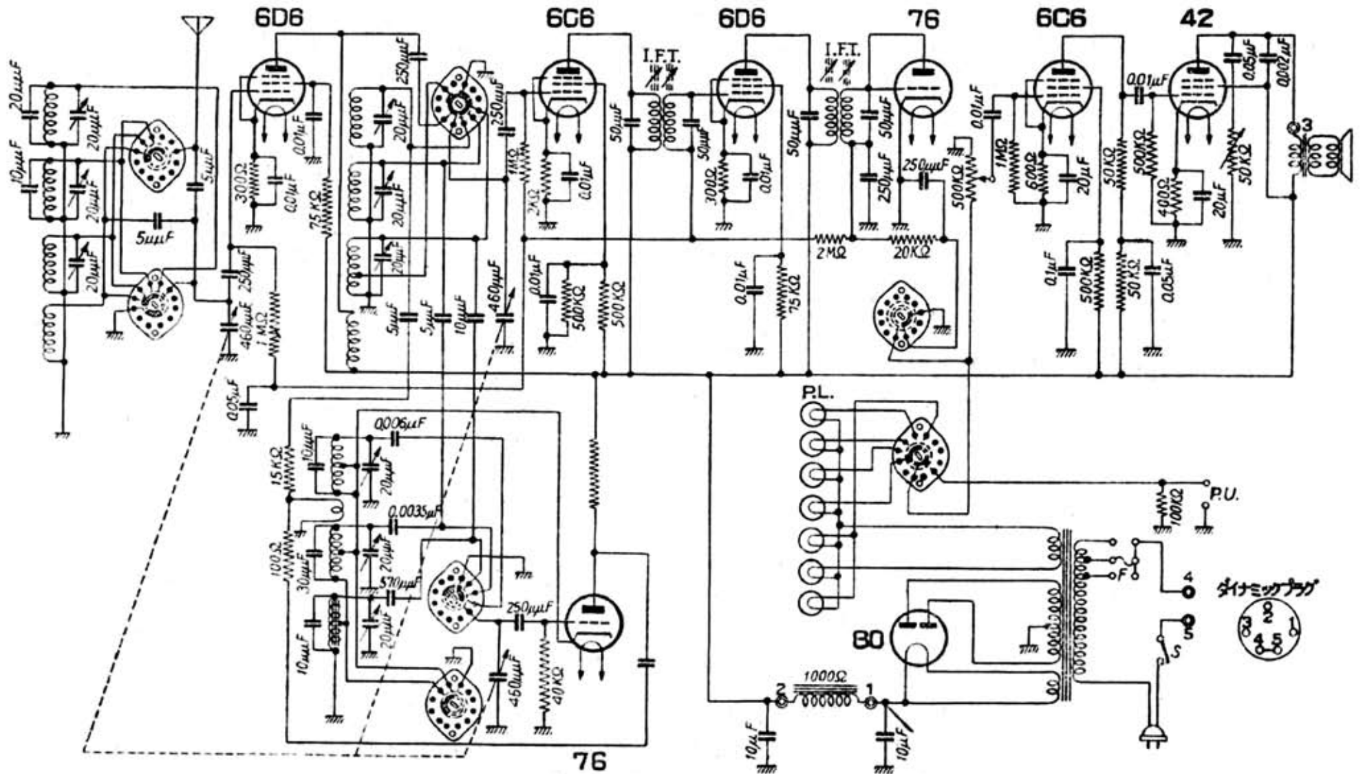
松下電器産業製 [ナショナルA-1型] 8球オールウェーブ受信機
