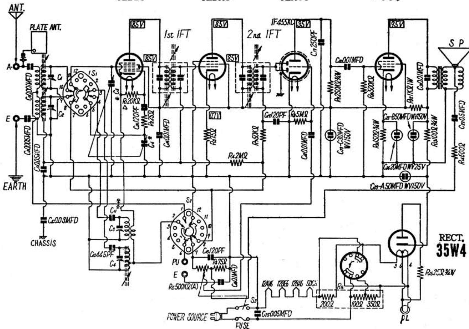
CONV. 12BE6
