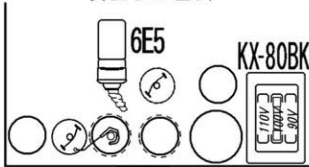
真空管配置図
